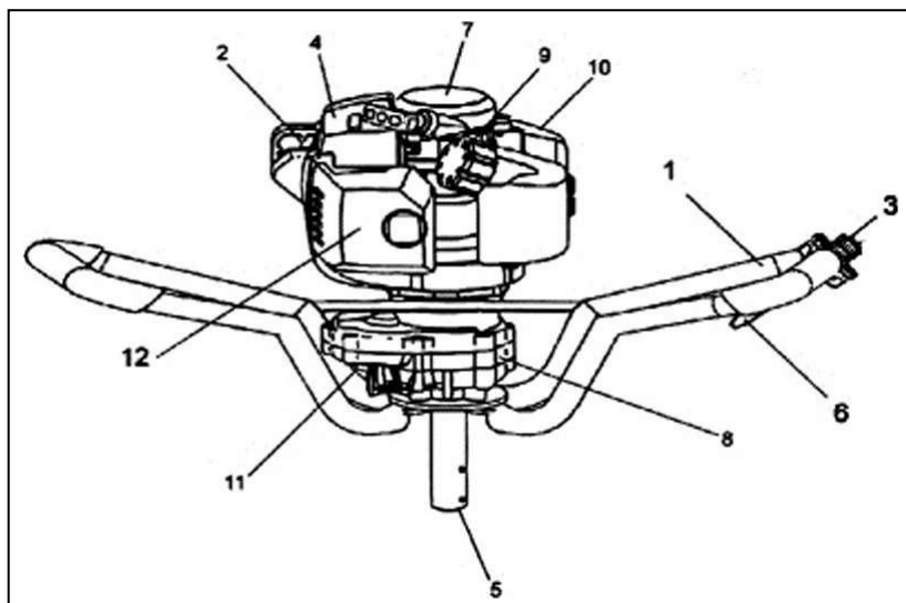
Рис. 1 Общий вид модели GGD-1,9/30RS
